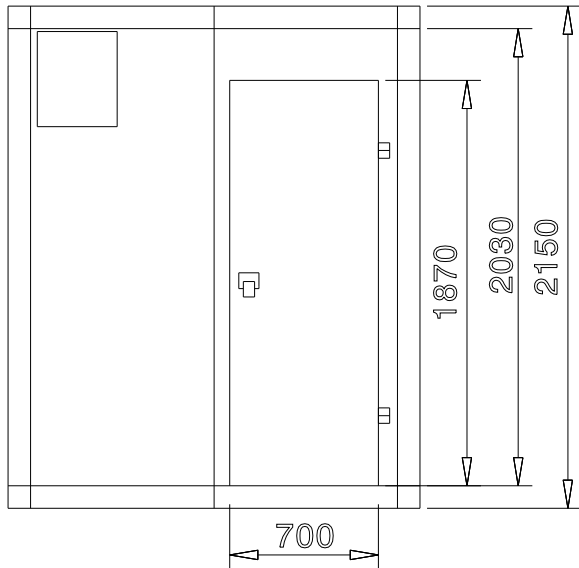
Zij aanzicht
